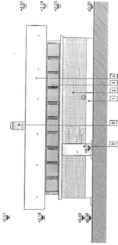
Meglévő észak-keleti homlokzat m 1:100
